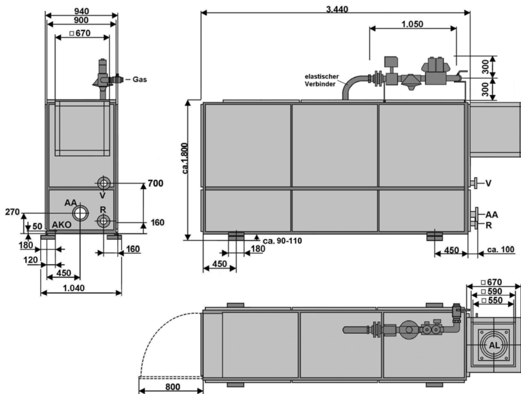
Abb. 5 Abmessungen und Anschlüsse der BHKW Module Vitobloc 200 BM-98/150 (MaÙe in mm); die bereits montierte Lüfterbox an der Rückseite kann für das Einbringen des Moduls demontiert werden
