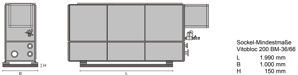
Abb. 7 BHKW mit Sockel
