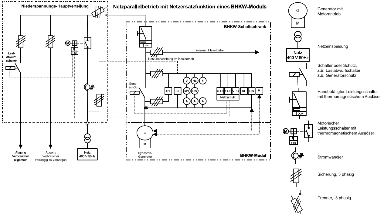
Abb. 4 Prinzipschaltbild der elektrischen Einbindung im Netzparallel- mit Netzersatzbetrieb
