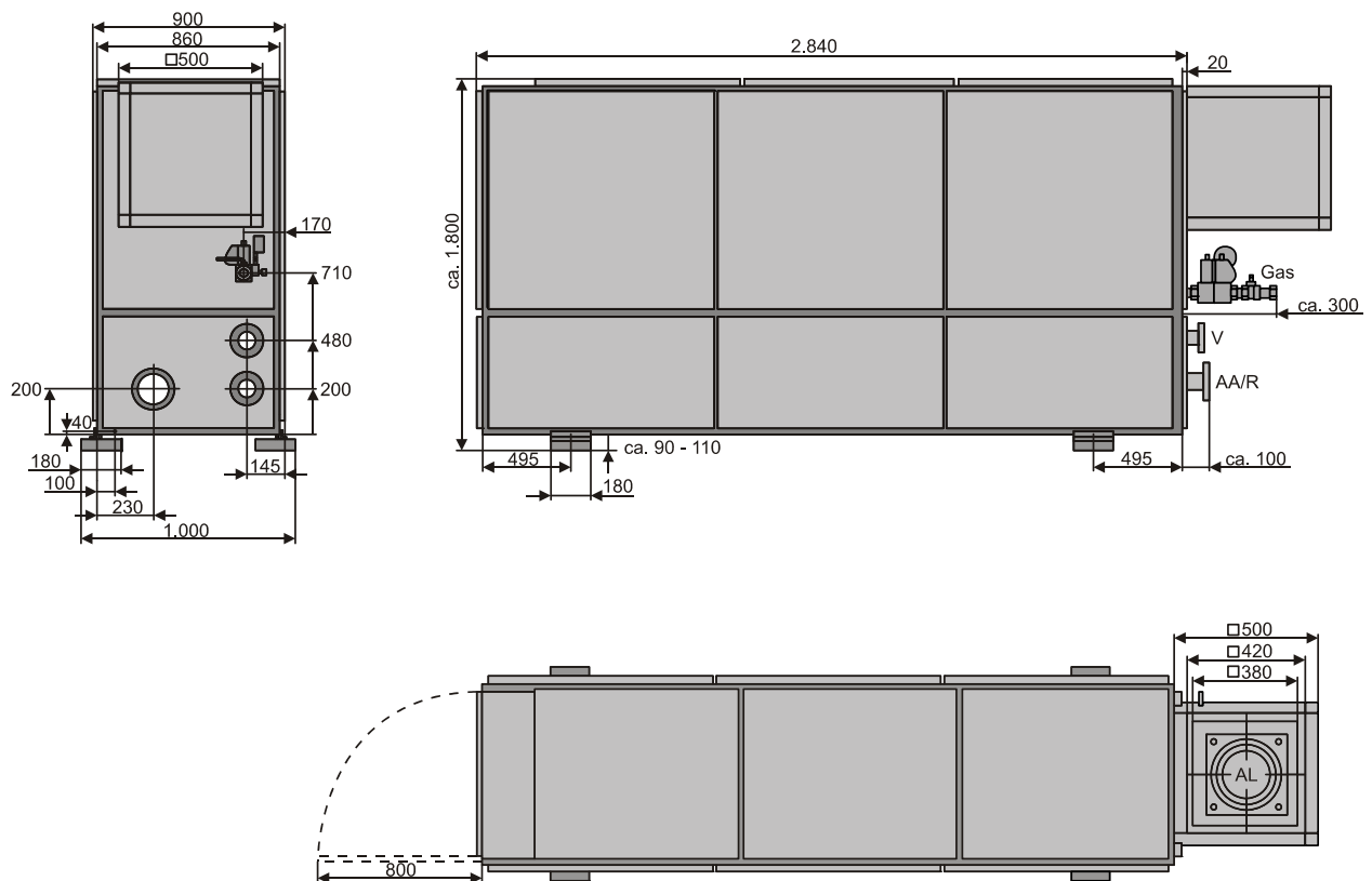
Abb. 5 Abmessungen und Anschlüsse der BHKW Module Vitobloc 200 BM-36/66 (Maße in mm); die bereits montierte Lüfterbox an der Rückseite kann für das Einbringen des Moduls demontiert werden
