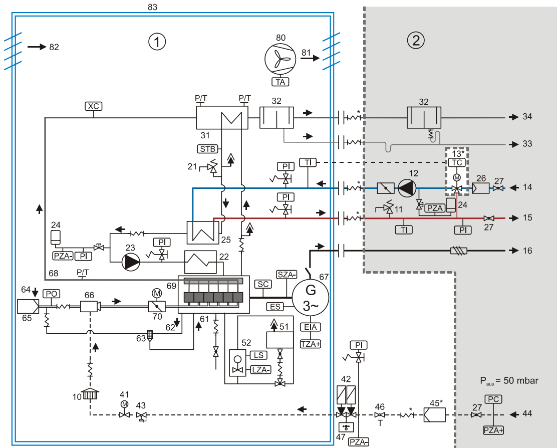
Abb. 2 Überwachungseinrichtungen
